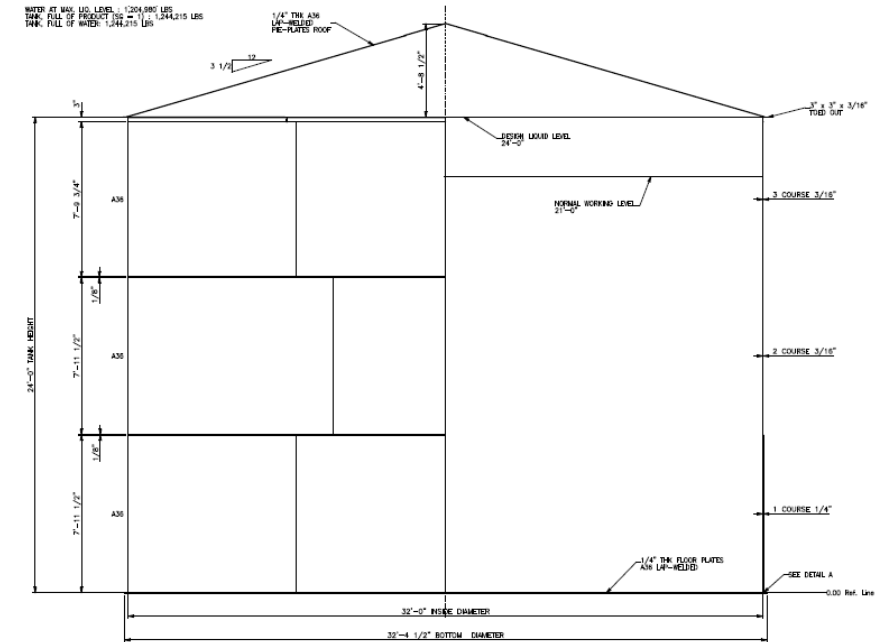
TES TANK DIAGRAM
